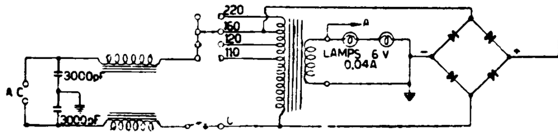
SICART-EMERSON - Mod. 803. Apparechio di minime dimensioni con sola gamma onde medie e con due finali in controfase. Media frequenza 455 kc/s. 3 watt di uscita.
